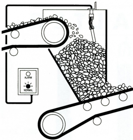
► Fallrohr oder Zwischenbunker Überfüllungsüberwachung
