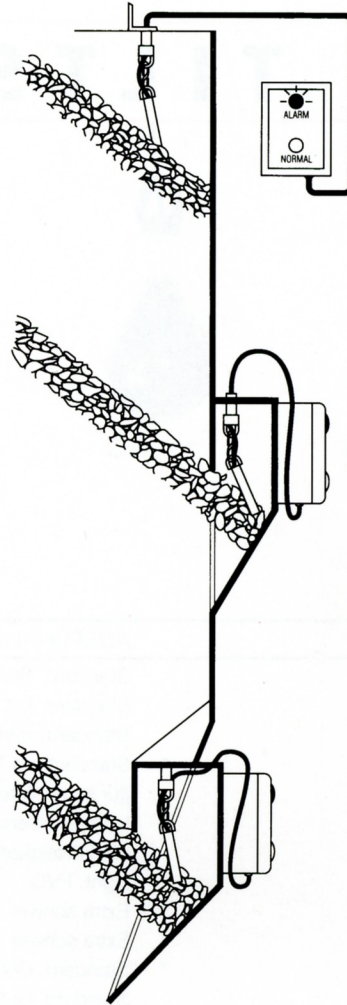
► Punktuelle Füllstandsüberwachung in Bunker und Silos
